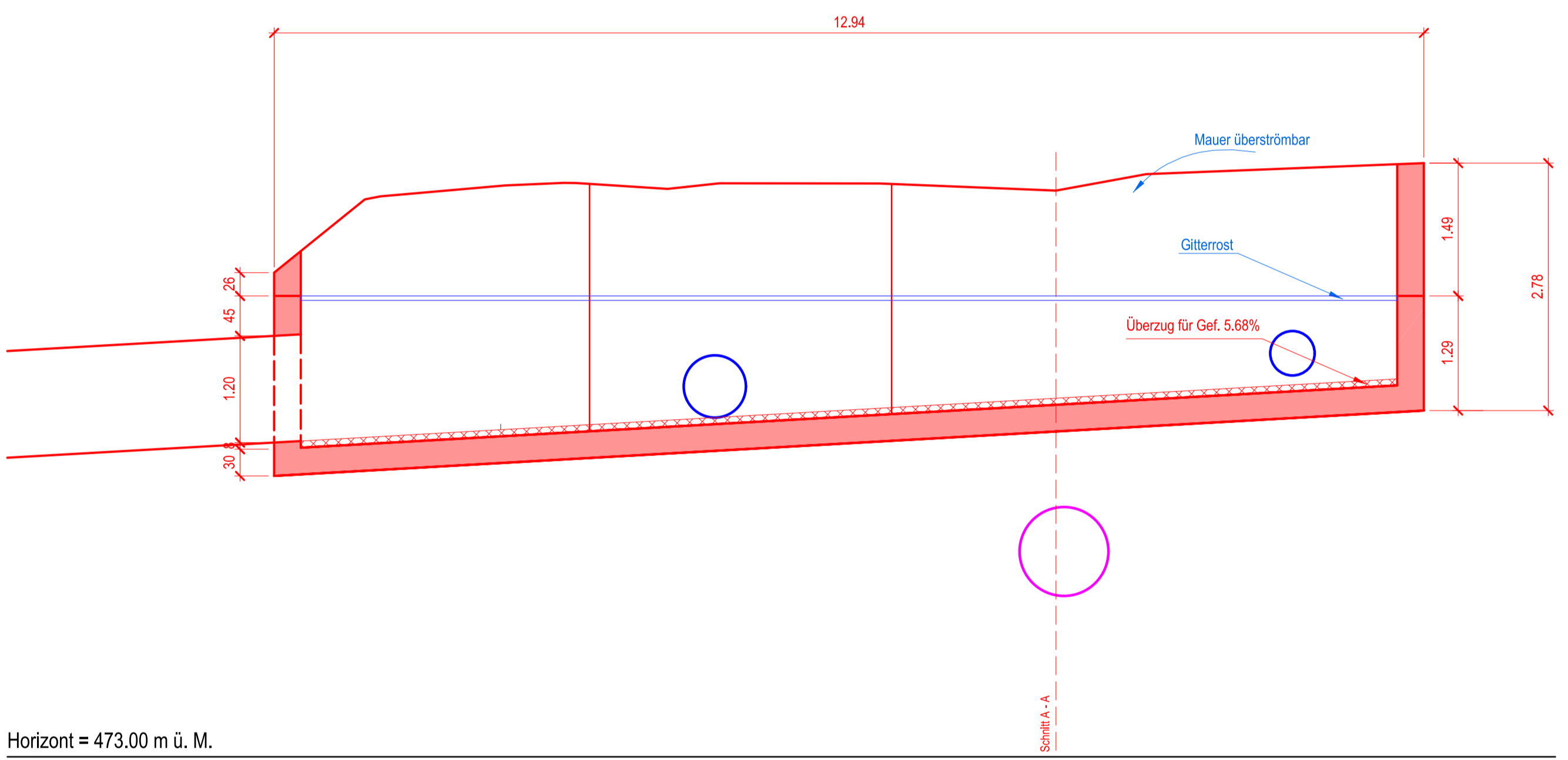
Einlaufbauwerk Schnitt B 1 : 50
