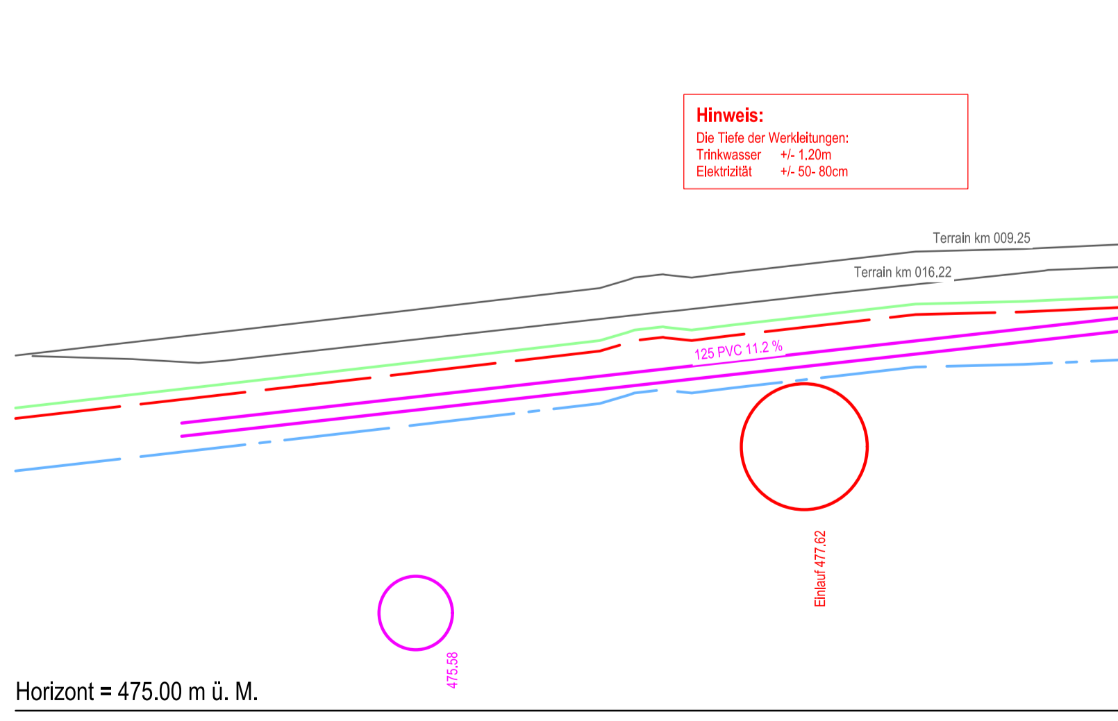
Einlaufbauwerk Schnitt C 1 : 50
