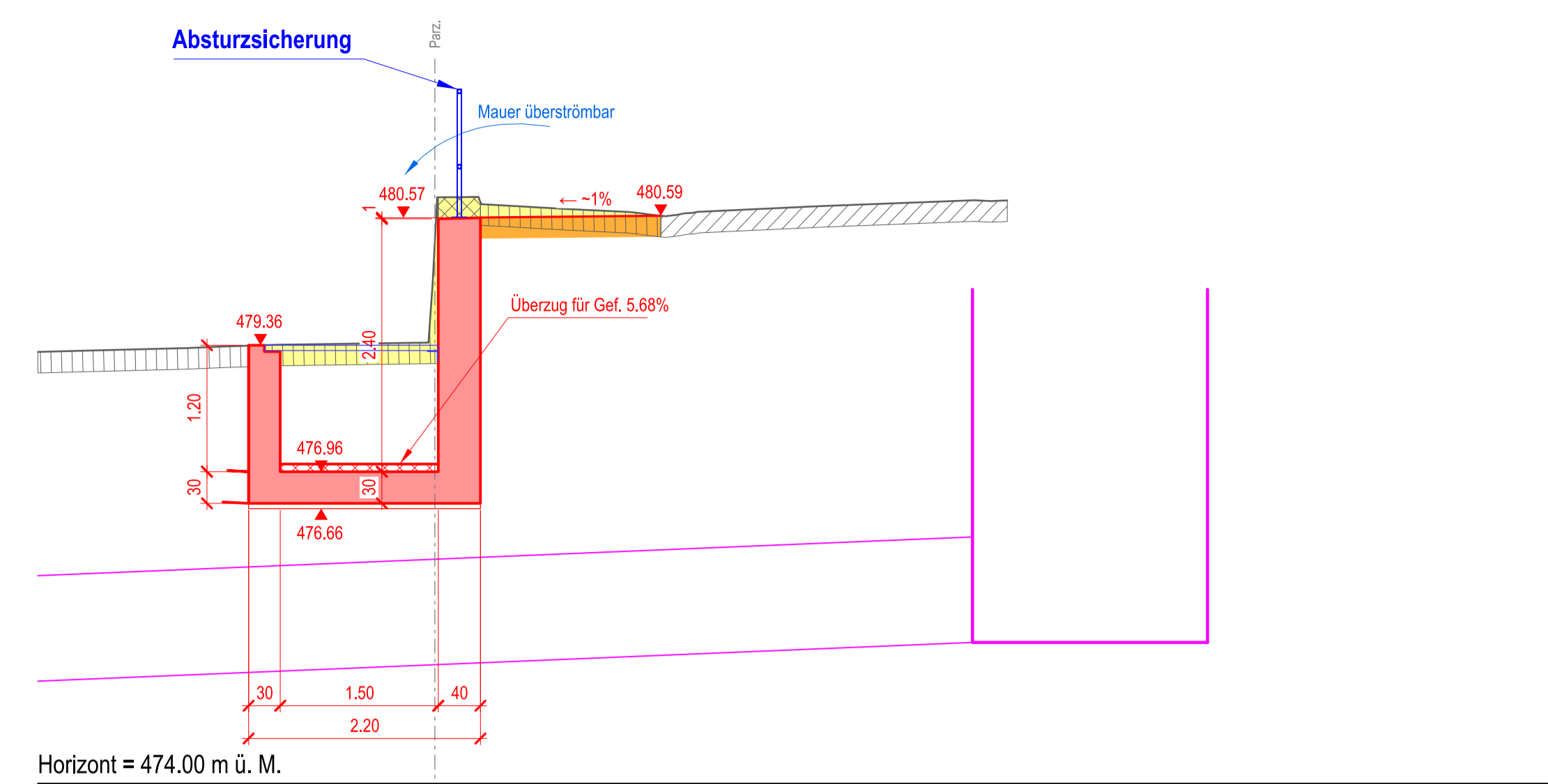
Einlaufbauwerk Schnitt A 1 : 50
